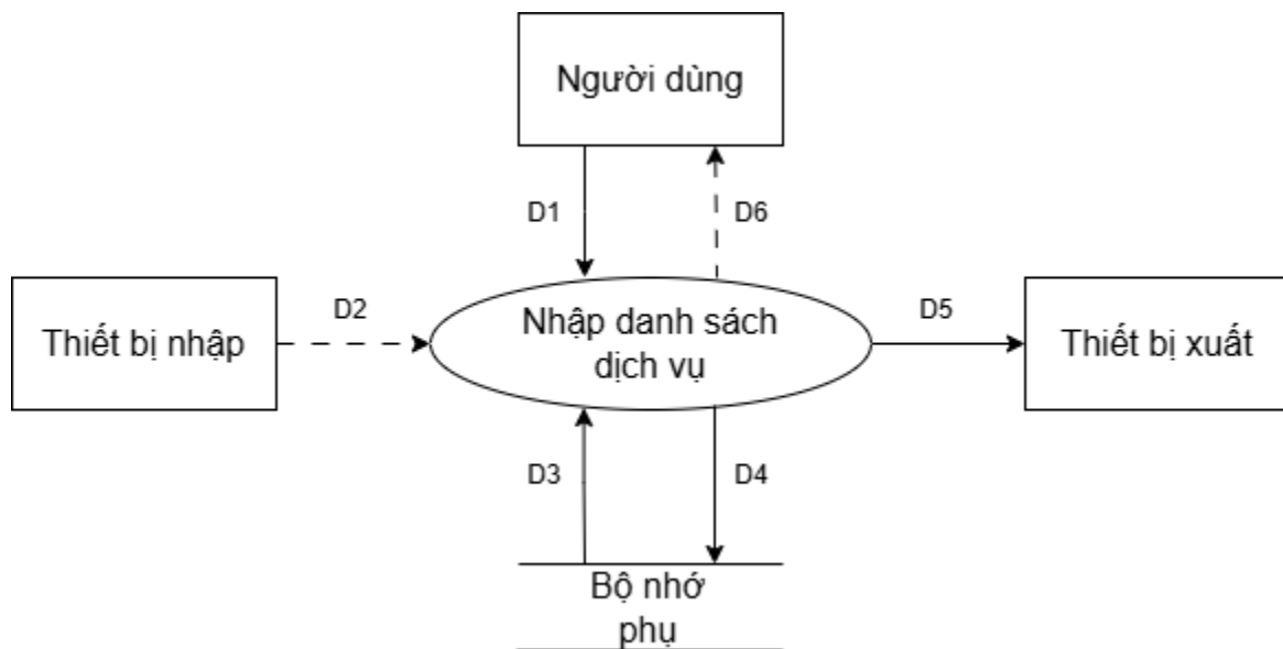
Sơ đồ DFD 6.3: Nhập danh sách dịch vụ
