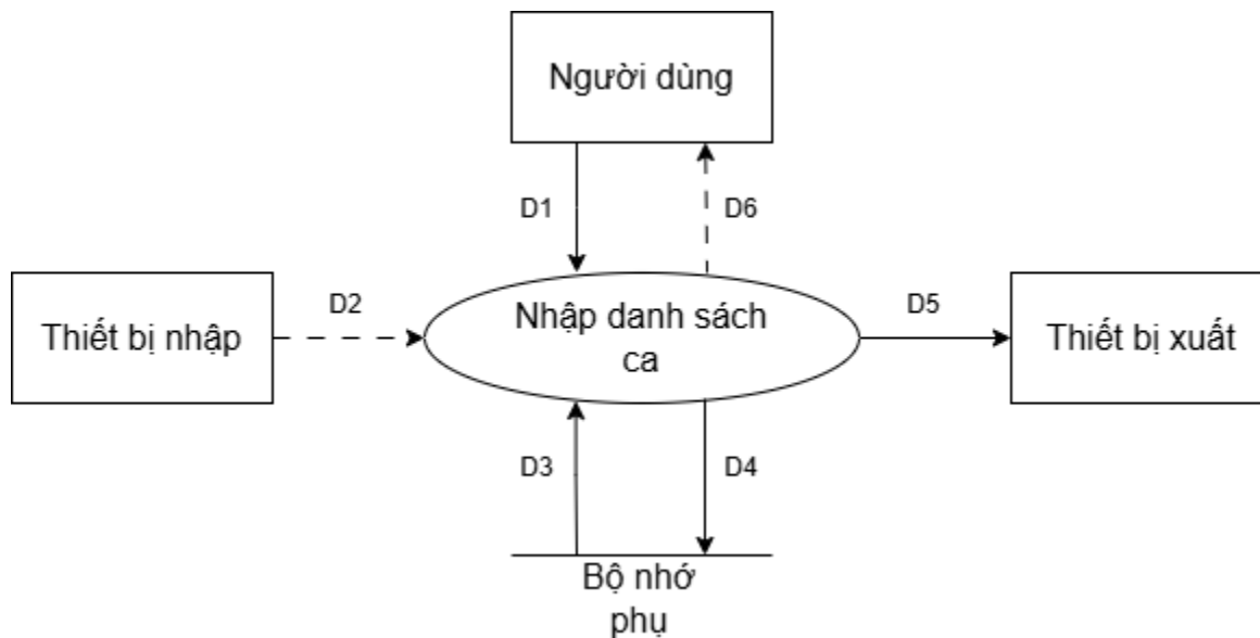
Sơ đồ DFD 6.2: Nhập danh sách ca
