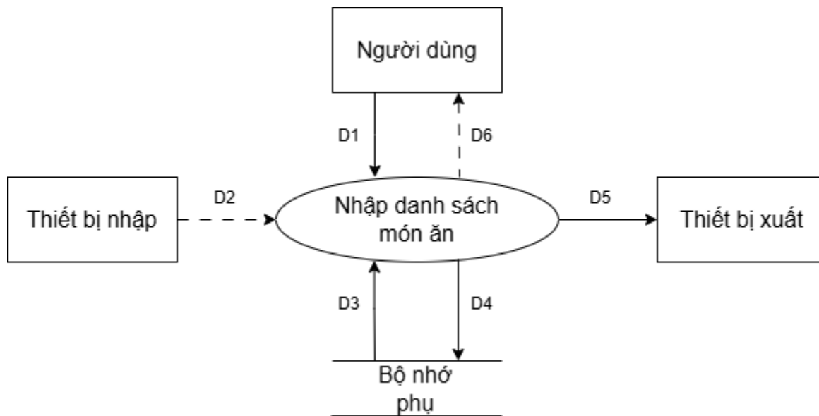
Sơ đồ DFD 6.4: Nhập danh sách món ăn
